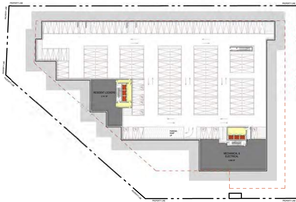
1 P2 A2.01 1:500
