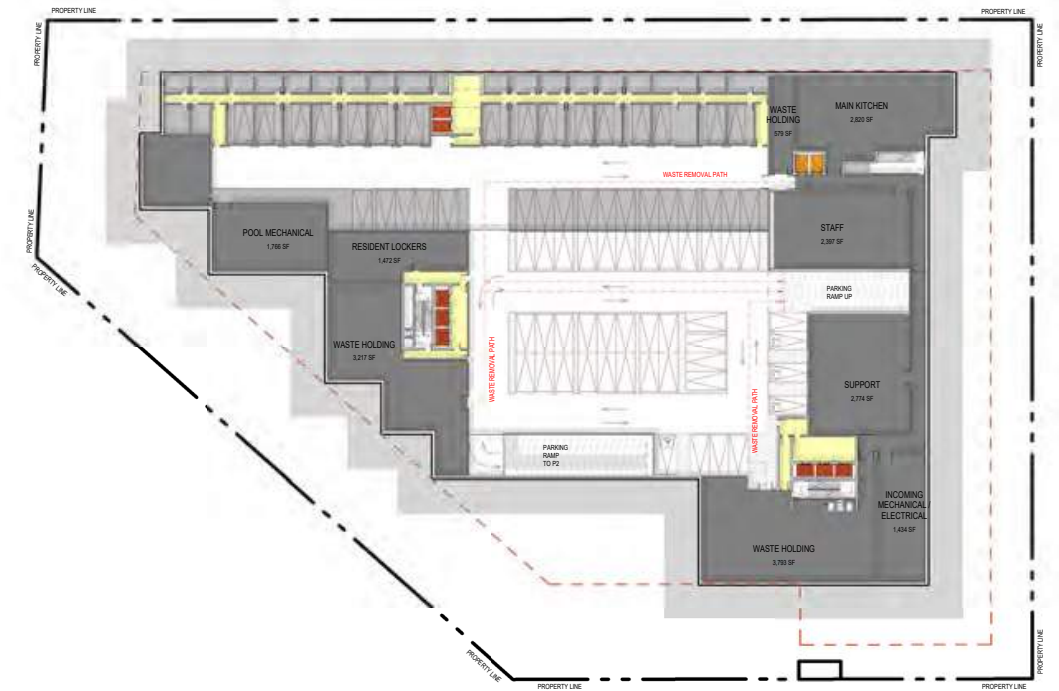
2 P1 A2.01 1:500
